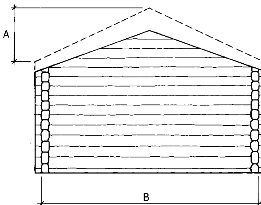
Figur 1. Takvinkelen endrer seg når bygget synker (fra Byggetaljer 523.291 Laftede vegger, fig. 314, © Norges byggforskningsinstitutt).
